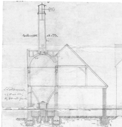
Gunzenhausen (Dld) 1881, bouwtekening 'hopfendarre'
